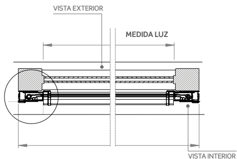
APL. ESTÁNDAR (FIG. 1)
