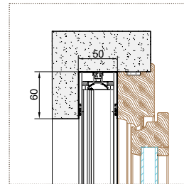
■ BORA INCAS ESTÁNDAR DOBLE 35/35
