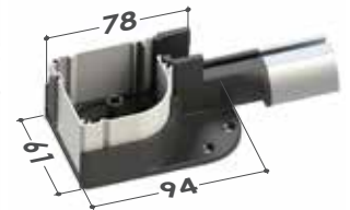
■ Cajón de 55 Cabezales inferiores
