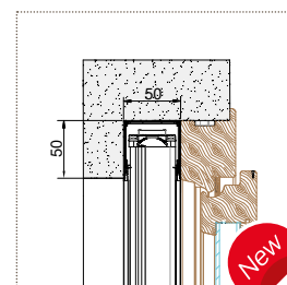
■ BORA INCAS MIDI DOBLE 50/50
