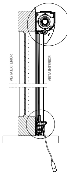
APL. ESTÁNDAR (FIG. 1)
