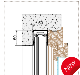
■ BORA INCAS MIDI DOBLE 35/35
