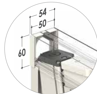
Cierre en bayoneta
