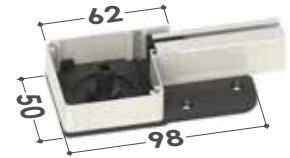
■ Cajón de 50 Cabezas inferiores
