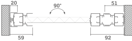
SECCIÓN HORIZONTAL 2 HOJAS A SEGUIR
