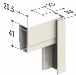
Guía telescópica regulable
