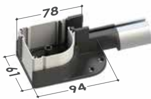
■ Cajón de 55 Cabezas inferiores
