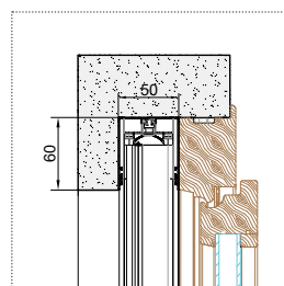
■ BORA INCAS ESTÁNDAR DOBLE 50/50
