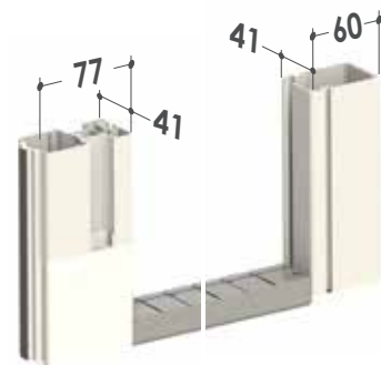
Cierre en bayoneta
