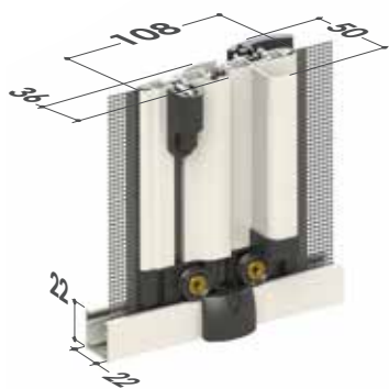
■ Barra manilla doble
