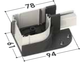
■ Cajón de 55 Cabezas inferiores
