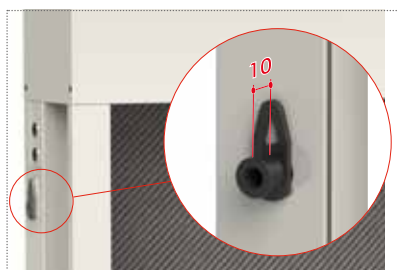
■ Guía con compensador completo de reglas: las reglas o registros de regulación , posicionados en las guías laterales, garantizan la instalación en huecos que no se cuadran o en presencia de superficies irregulares y no homogéneas. Regla de compensación hasta 10 mm .
