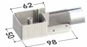
■ Cajón de 50 Cabezales inferiores
